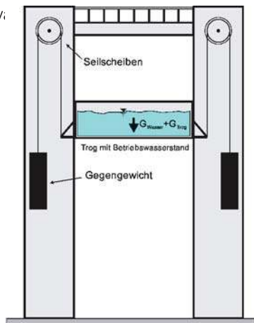
Bild 4: Funktionsprinzip des Hebwerks in Scharnebeck
